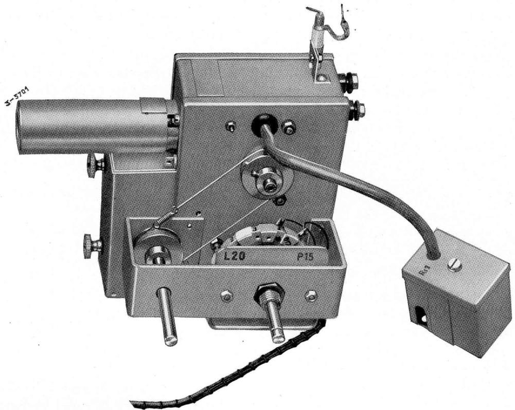
Abb. 10. Baustein Quarzoszillator (3) für nachträglichen Einbau
