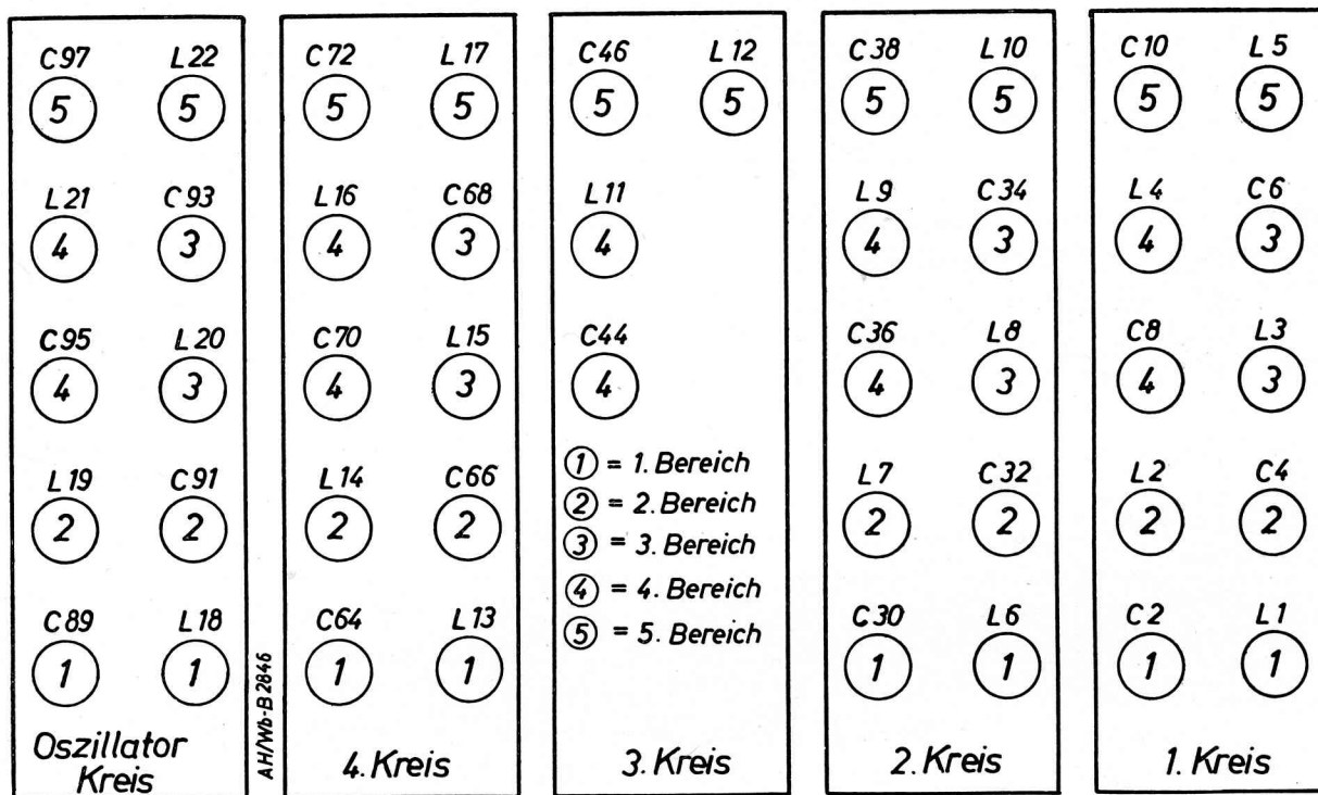
Abb. 7. HF-Teil (1) Abgleichplan der 5 Bereiche
