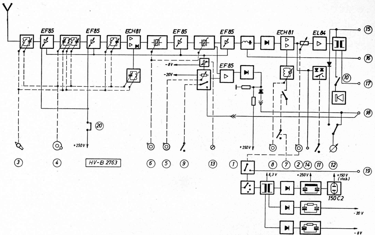
Abb. 2. Blockschaltbild des Kw-Empfängers E 127 Kw/4
