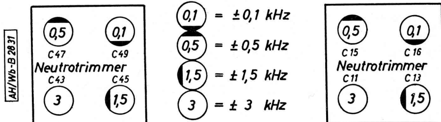
Lage der Neutro-Trimmer
