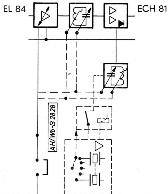
Abb. 11. Blockschaltbild des Quarzoszillators mit 6 wählbaren Quarzen
