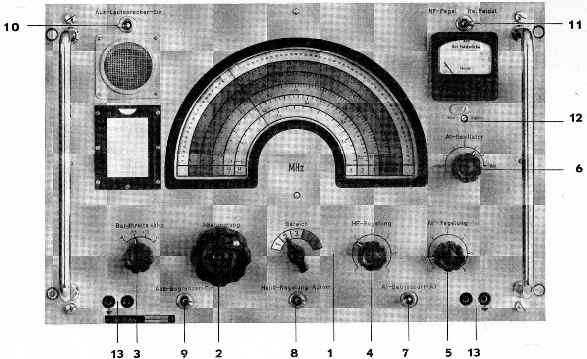
Abb. 4. Frontplatte des Kw-Empfängers E127 Kw/4
