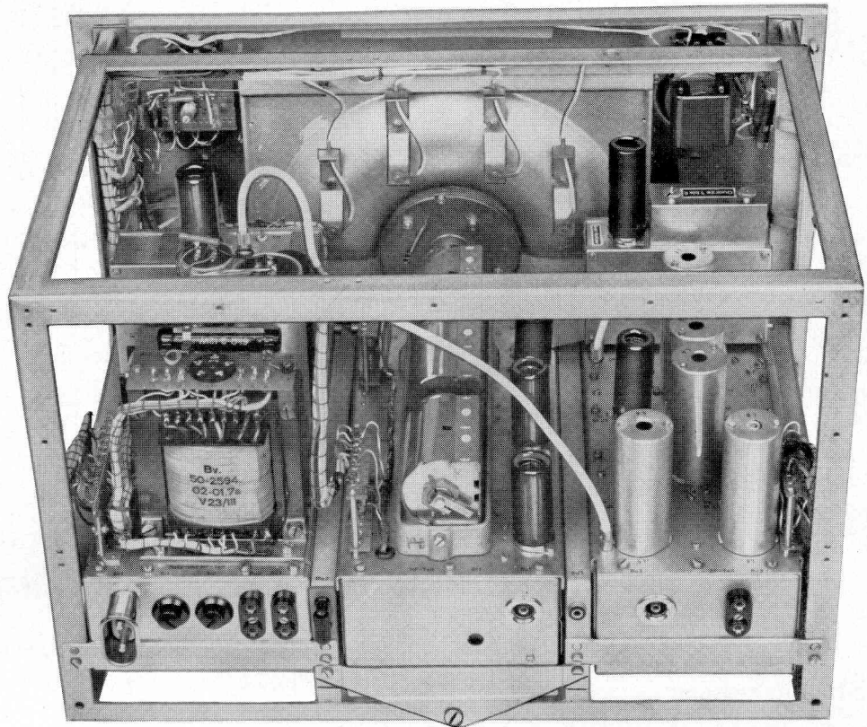
Abb. 3. Rückansicht des Kw-Empfängers E127 Kw/4 ohne Gehäuse
